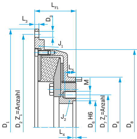
Abb. 1: keine Durchdrehsicherung
