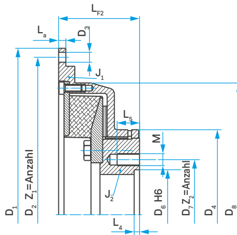
Abb. 1: mit Durchdrehsicherung
