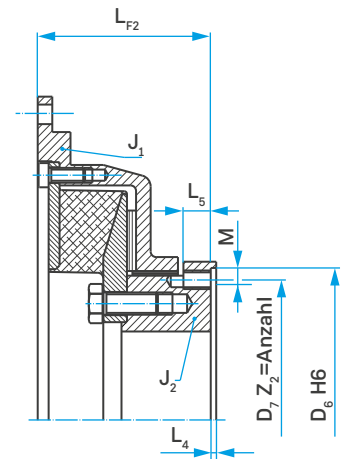
Abb.2: keine Durchdrehsicherung
